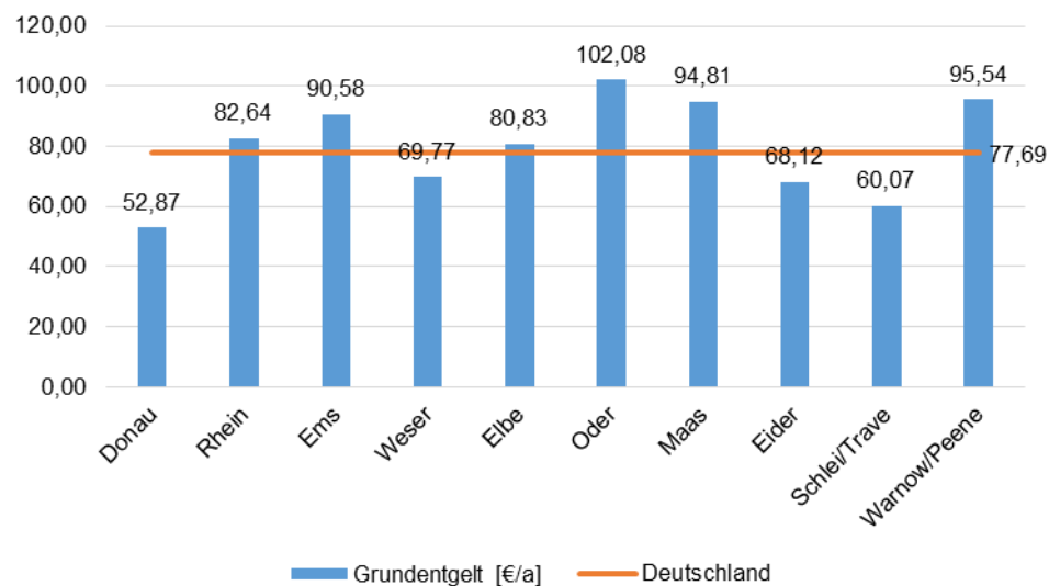
Abbildung 3-14: Trinkwassergrundentsgelte alle FGE (Bruttoentsgelte auf der Basis von nach Einwohnern gewichteten Gemeindedaten, Zuordnung der Gemeinden nach dem qualifizierten Leitband, Stand 2016)
