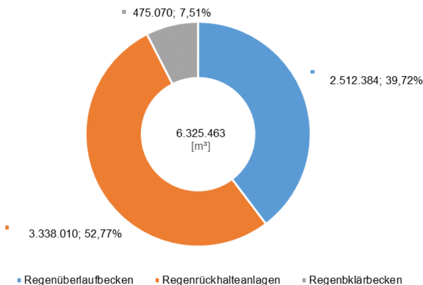
Abbildung 3-23: Speichervolumen der Regentlastungsbauwerke FGE Donau (Stand 2016)
